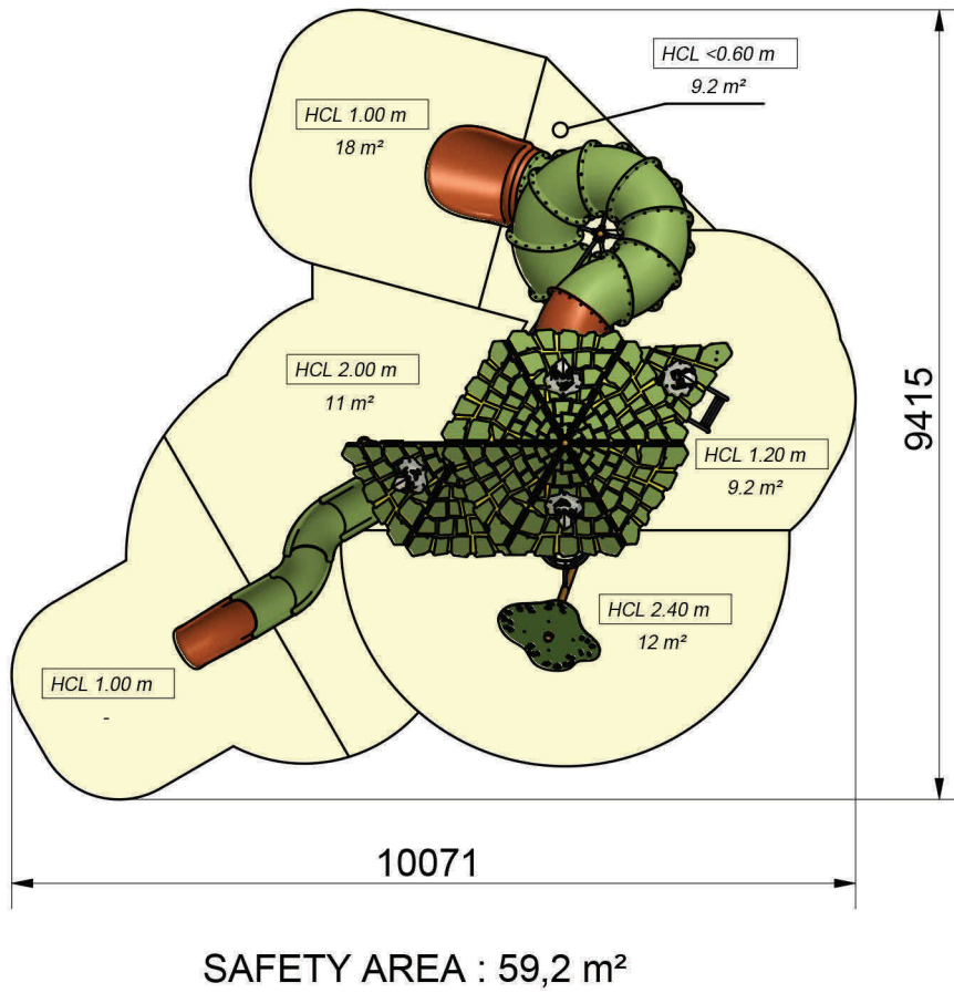
Vue du dessus et coupe à l'échelle 1/100
